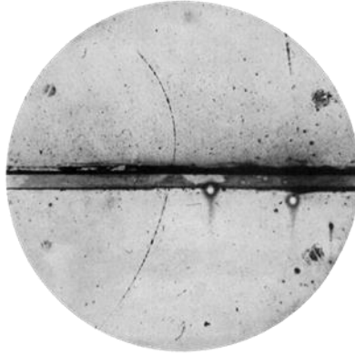
أول صورة مأخوذة للبوزيترون في ثلاثينيات القرن العشرين
