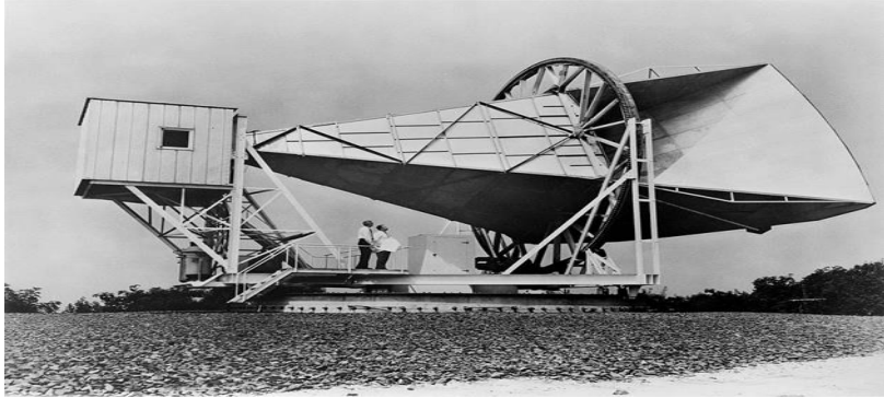
الهوائي المركب الذي التقط الأشعة الكونية لأول مرة في التاريخ
