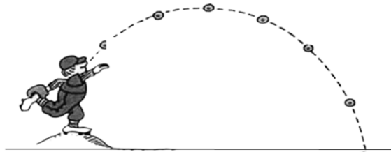
تسارع الحركة بمرور الوقت ليصل إلى الذروة
