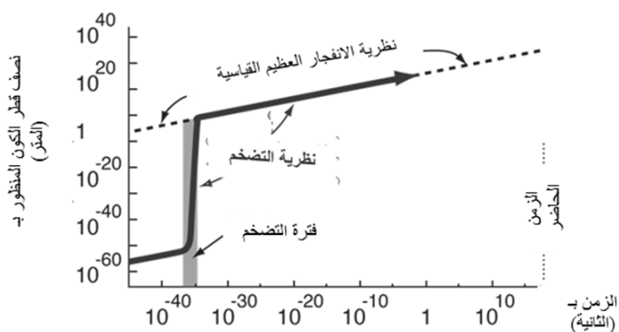
مخطط بياني لنموذج نظرية التضخم
