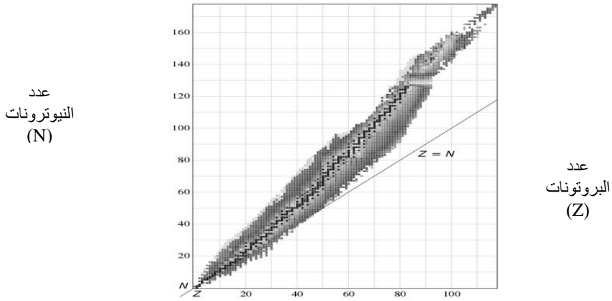
"جزيرة الاستقرار" لنظائر العناصر الكيميائية
