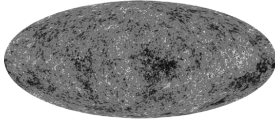
صورة حرارية للكون المرئي التقطها مسبار ويلكيנסون
